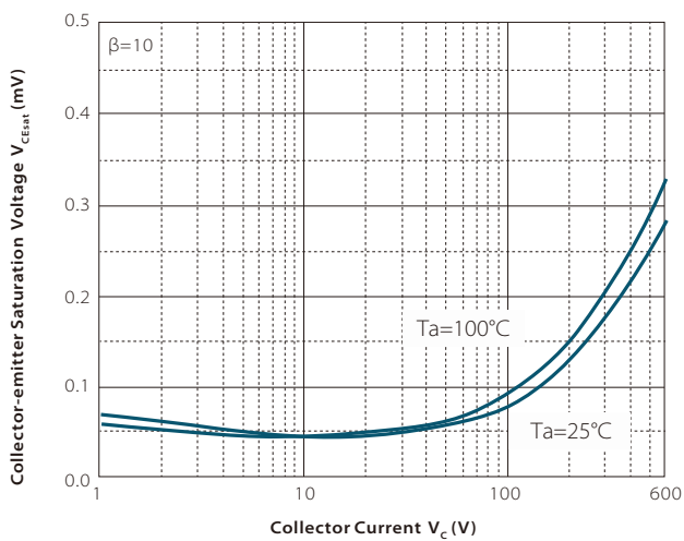
V_{CE\text{sat}} \text{ — } I_C
