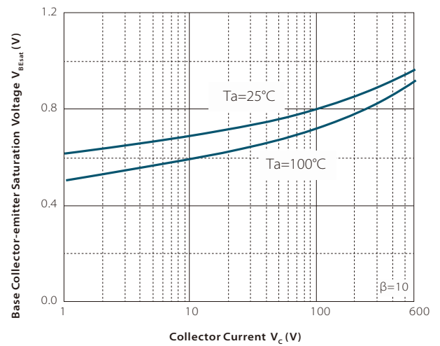
V_{BE\text{sat}} \text{ — } I_C
