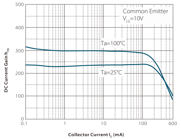
h_{FE} \text{ — } I_C
